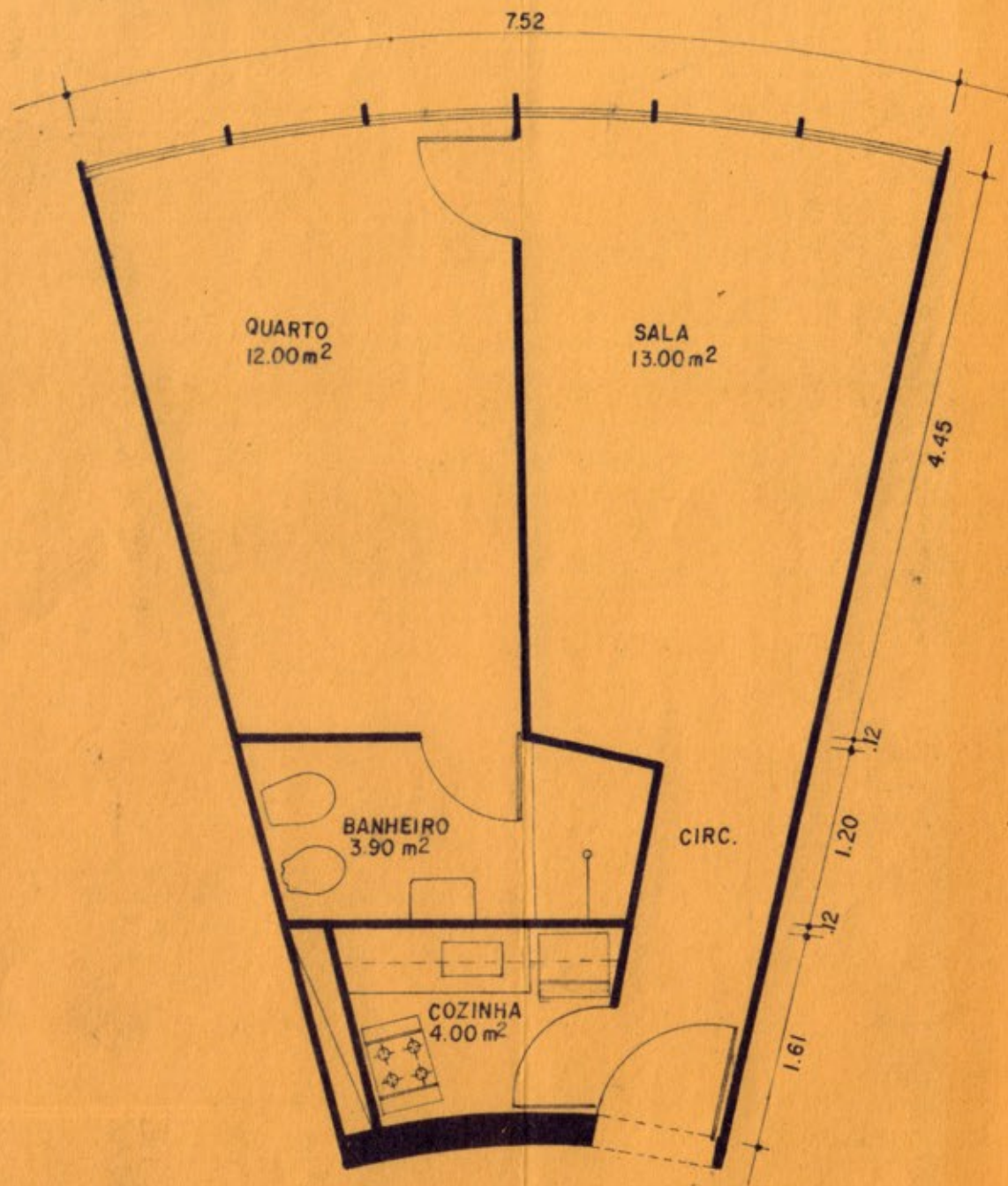
PLANTA BAIXA DO APARTAMENTO ESC. 1:50
